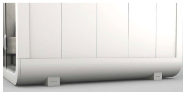
GummifüÙe zur Schall-Abkopplung der Kabine vom Boden. 8mm Luft zwischen Boden und Kabine
