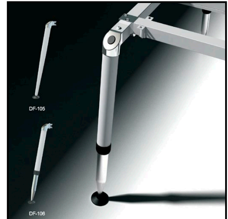
Bench design mit höhenstellbaren Füßen (Gestellalternative)
